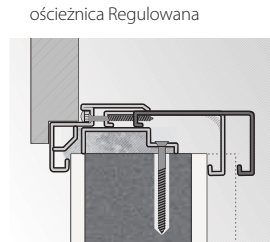
ościeżnica Regulowana
