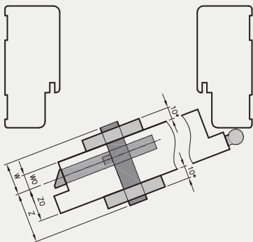
Rys. Dobór wymiaru wkładki bębnekowej
