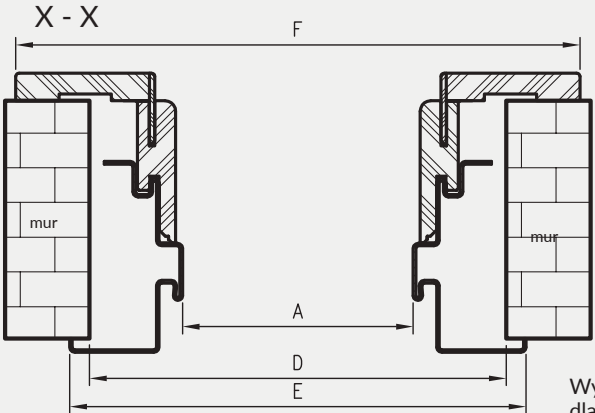
Profil ościeżnicy
