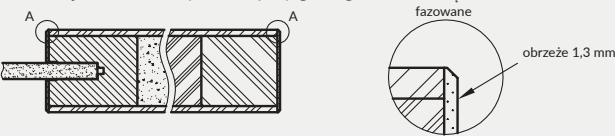
Przekrój ramia skrzydła bezprzylgowego
