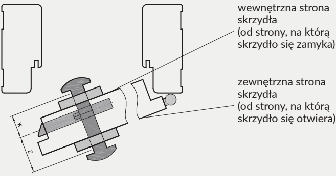
Rys. Dobór wymiaru wkładki z gałką
