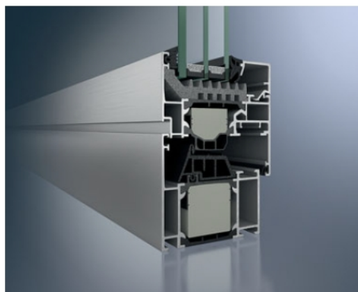
Schüco AWS 75.SI+ Standardowy kontur o izolacyjności cieplnej odpowiadającej aktualnym wymaganiom
