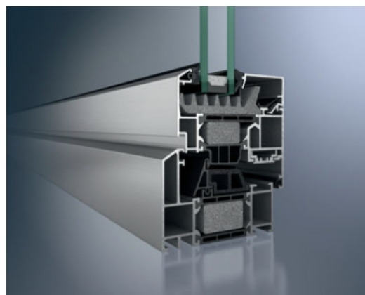
Schüco AWS 75 RL.SI+ Wyjątkowy kontur, szczególnie zalecany przy modernizacji i dla podkreślenia indywidualnego stylu
