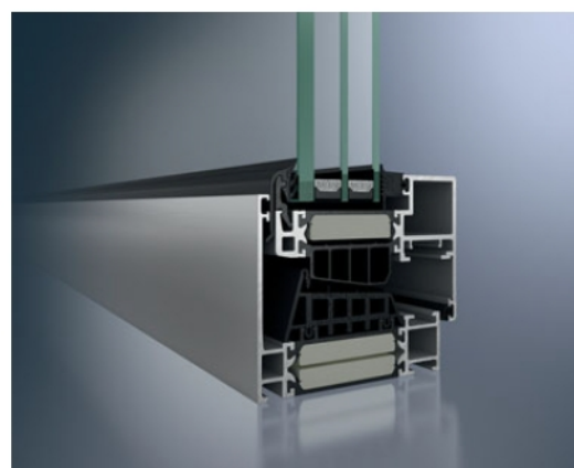
Schüco AWS 90 BS.SI+ Minimalistyczny kontur okna z ukrytym skrzydłem
