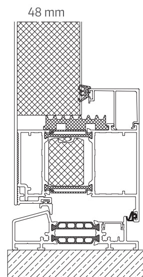
Aliplast STAR 90 mm
