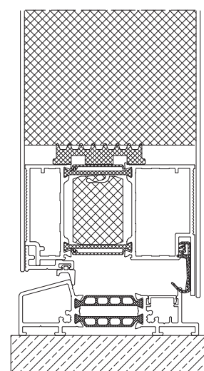
Aliplast STAR 90 mm
