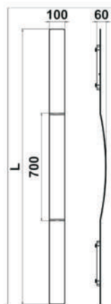
Uchwyt PS-W
