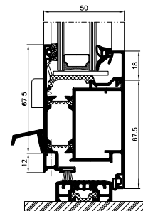
przekrój przez poprzeczkę dolną drzwi
