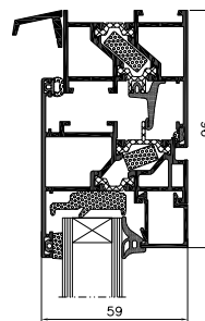
przekrój okna otwieranego na zewnątrz
