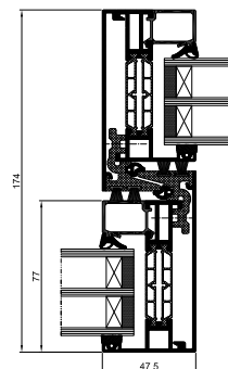
przekrój przez skrzydła drzwi
