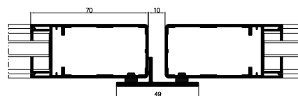
przekrój poziomy skrzydła z przyłągą
