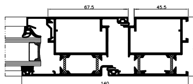
przekrój drzwi
