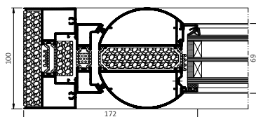
Przekrój przez bok drzwi (SI) z bezpiecznym przamykiem
