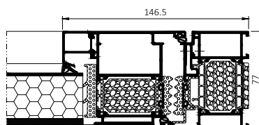
przekrój przez drzwi panelowe MB-86N SI+ w zabudowie witrynowej
