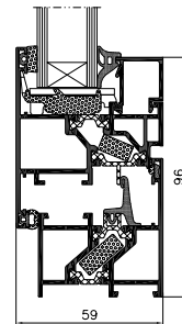
przekrój okna otwieranego na zewnątrz
