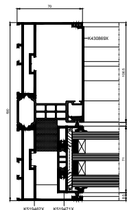
przekrój boczny drzwi
