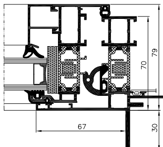
przekrój przez okno MB-70US
