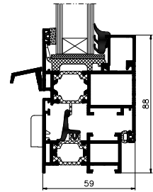
przekrój okna otwieranego
