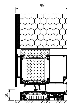
przekrój przez próg drzwi panelowych MB-104 PASSIVE Aero
